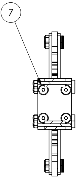
SECTION D-D
